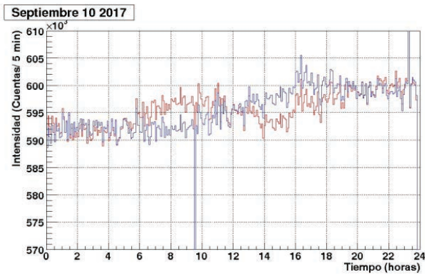
Figure 4: Registro de la fulguración solar Del 20170910 por el Monitor de Neutrones (MN) del Observatorio de Rayos Cósmicos de Chacaltaya (OR- CCh) con una resolución promedio de cuentas cada 5 minutos. Línea azul eventos de neutrones, línea roja registro de la presión en el observatorio para corregir datos.
